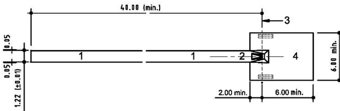
Dráha pro skok o tyči, rozměry v [m]
