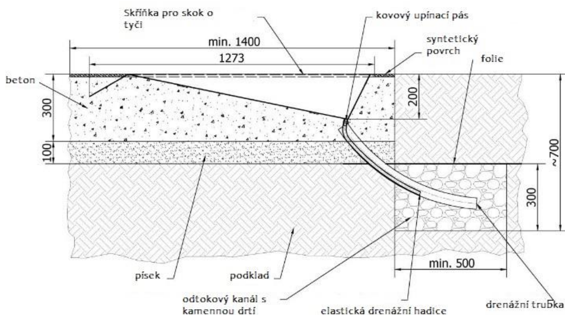
PVBOX-S instalovaný na dráze, rozměry v [mm]
