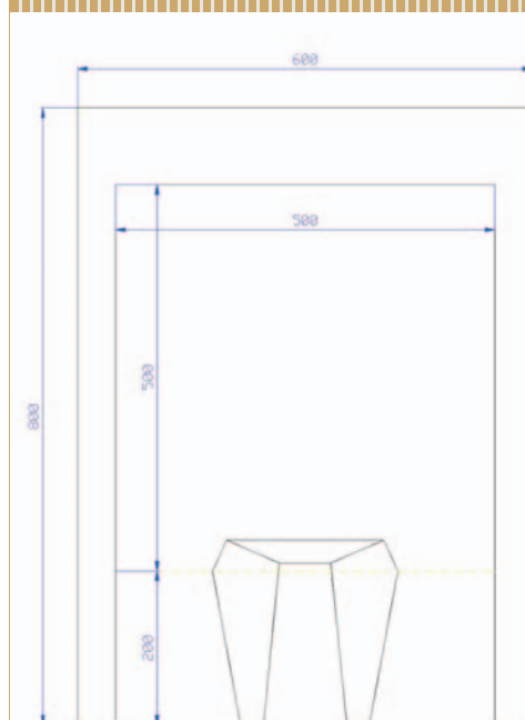
Schéma mimimální rozměry doskočiště
